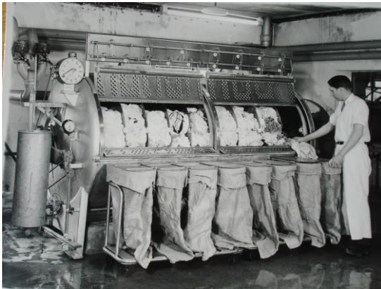
16 rums 200 kg, Veta vaskemaskine
